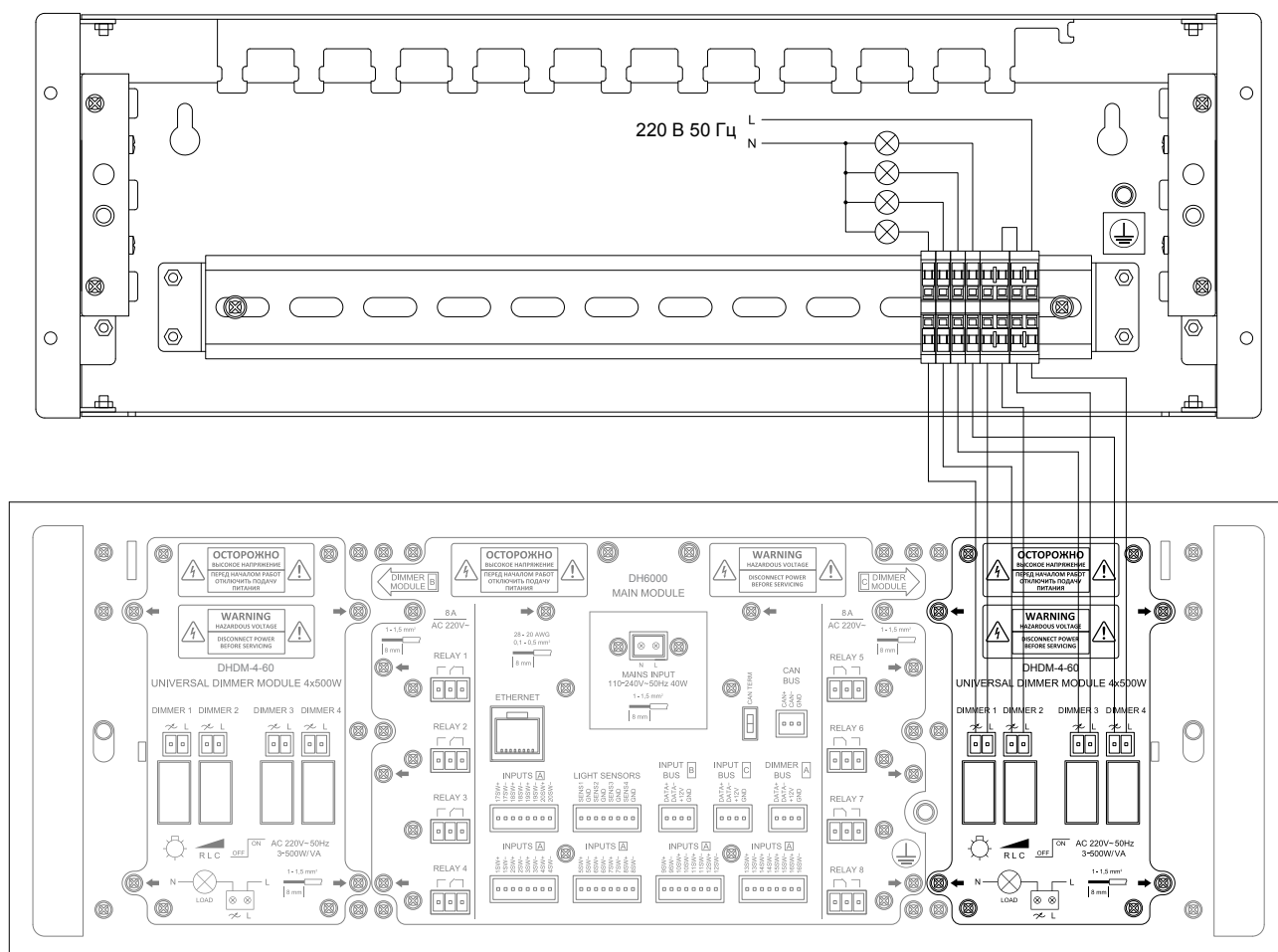
Рис. 1. Схема подключения модуля универсальных диммеров DHDM-4-60
